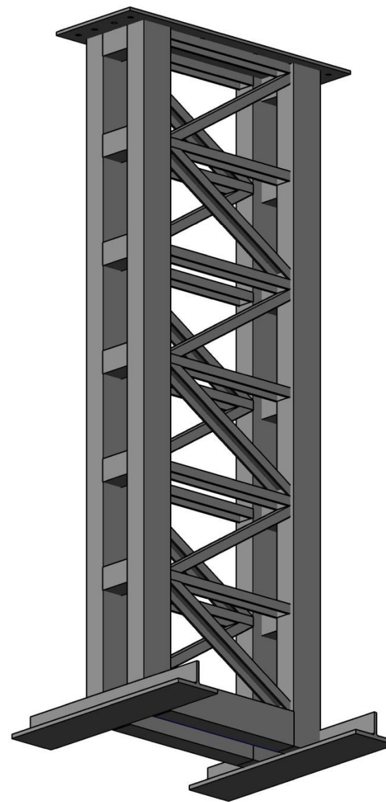
Nesošās kolonas konstrukcijas, principiālā shēma.
