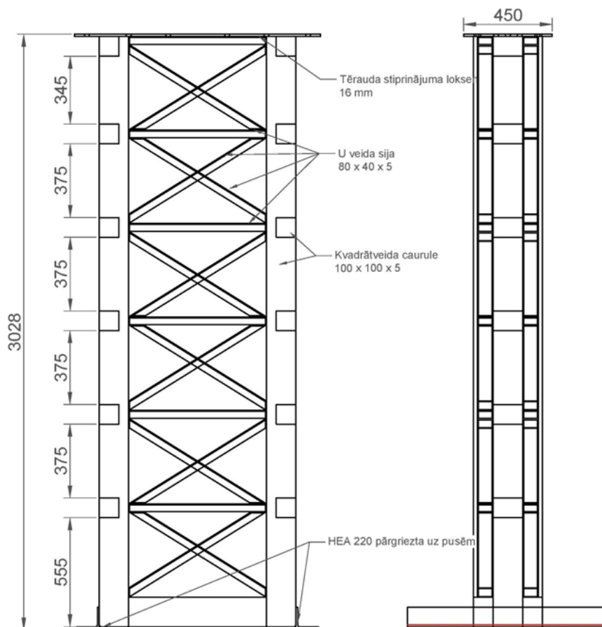
Augšējās konstrukcijas, principiālā shēma.
